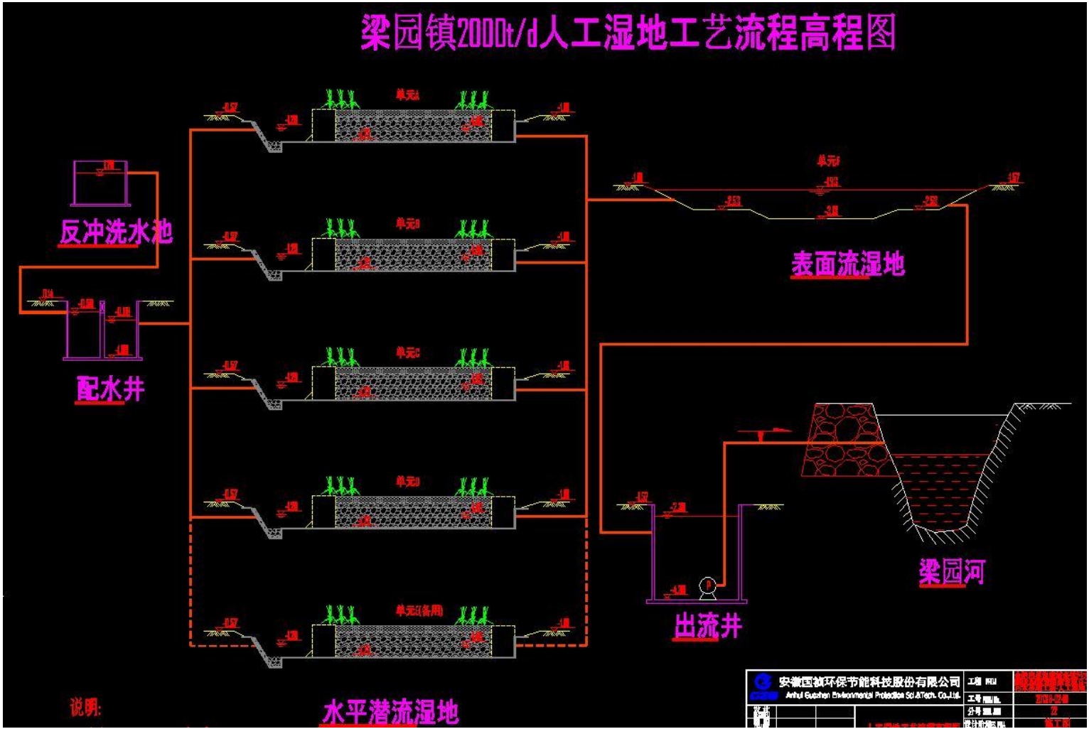
附件 4 项目工艺高程图
