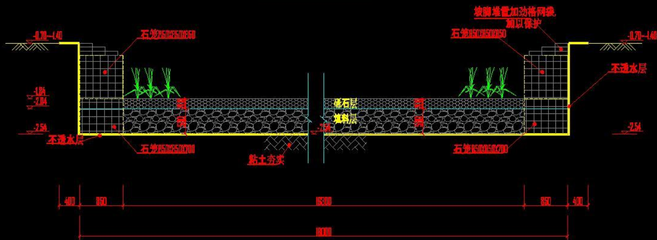
单元A、C、D II-II剖面图
