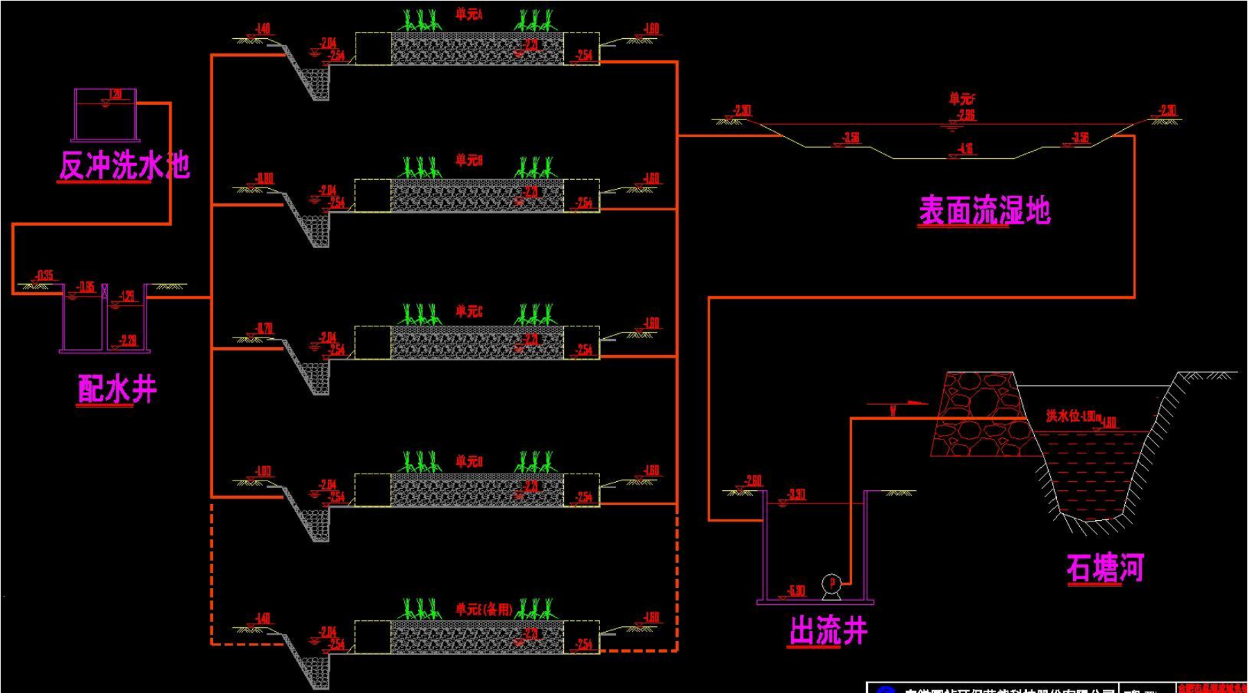
附件 4 项目工艺高程图
